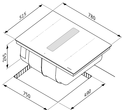
Abysso Down Air - 034062201
