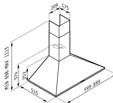
Square Chimney Plus 60cm - 065038001 Square Chimney Plus 90cm - 065037901
