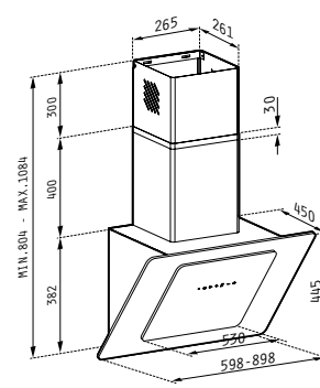
Fiero White Glass 60cm - 065023301 Fiero White Glass 90cm - 065023201
